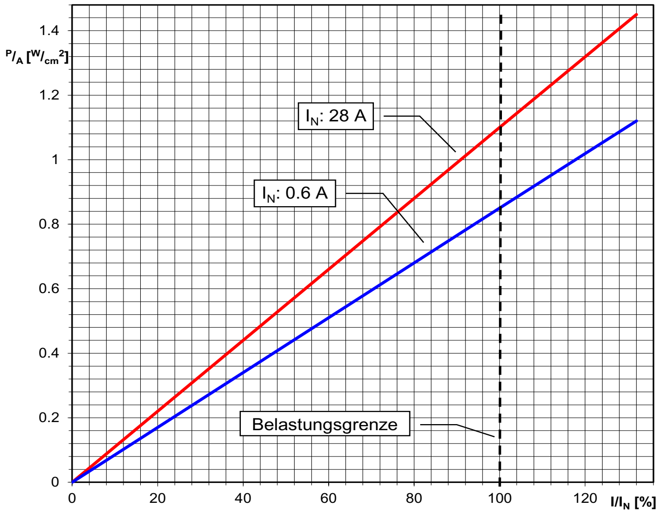
Oberflächenbelastung in Funktion der Belastung
