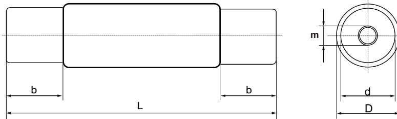
Gedrehte Kappen, Messing vernickelt Machined ferrules, brass, nickel-plating Bagues décollétées et taraudées, laiton nickelage
